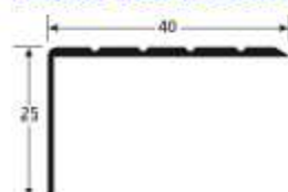
HOEKPROFIEL 40 x 25
