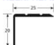
HOEKPROFIEL 25 x 20
