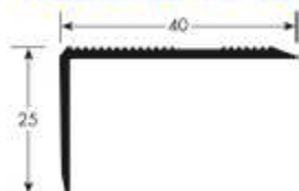
HOEKPROFIEL 40 x 25
